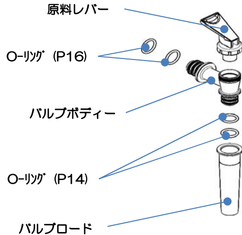
＜原料タンク弁の構成＞
