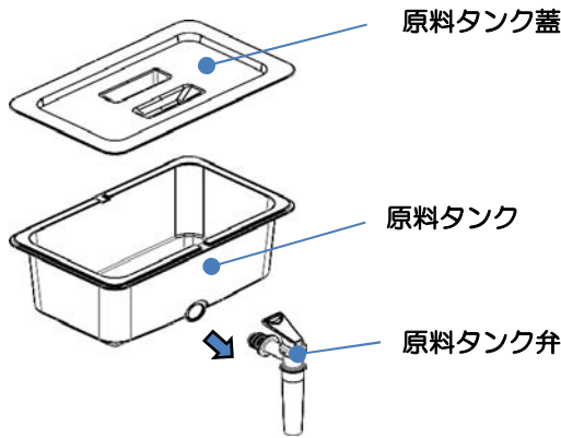
＜原料タンクの構成＞
